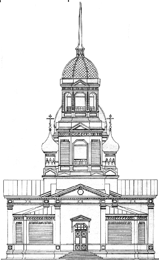
Проект на постройку деревянной церкви для Троицко-Сергиевского полка. Западный фасад. [1913 г.] ГАПО. Ф. 35. Оп. 1. Д. 330. Л. 2.
